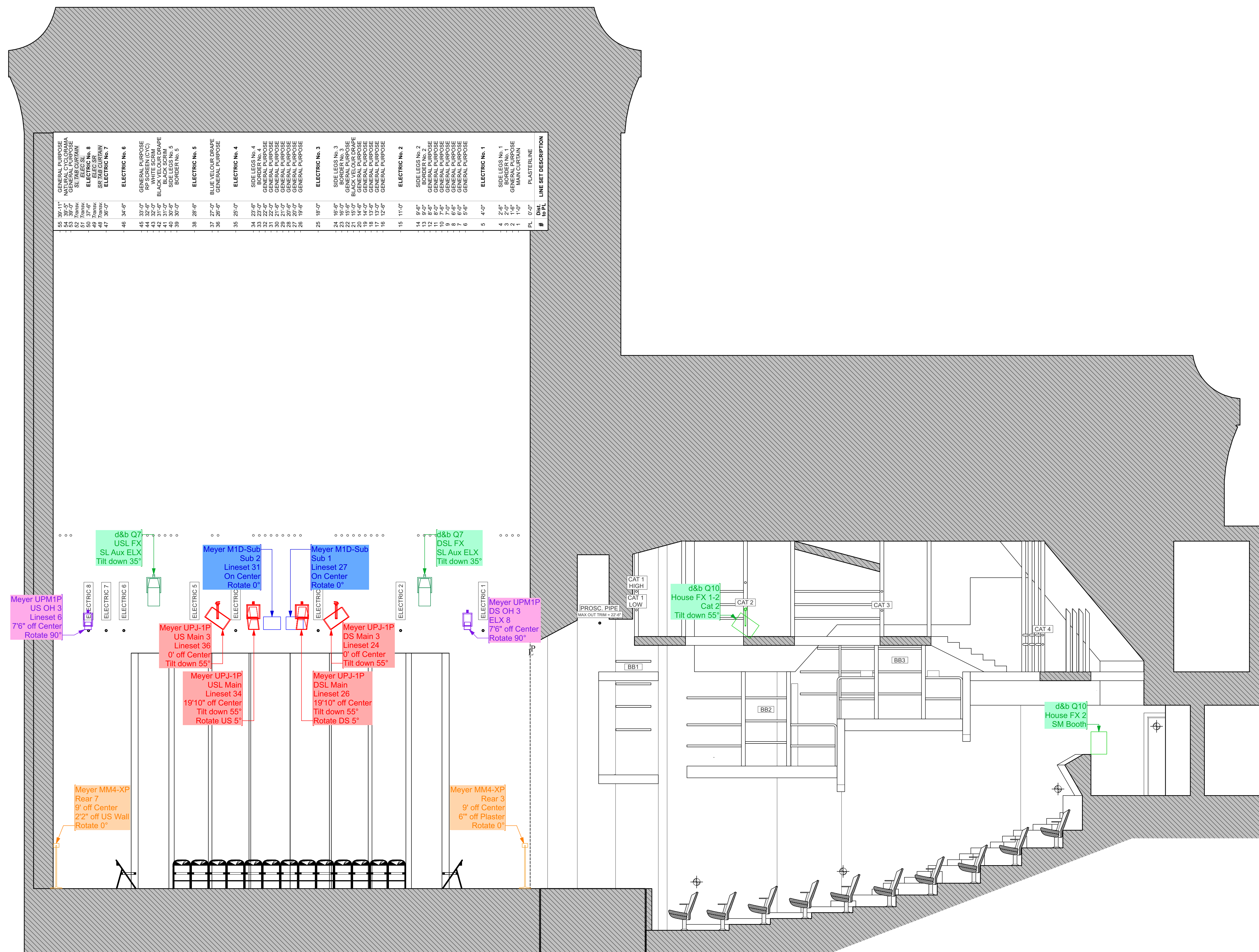
3 Section SL Scale: 1/4" = 1'-0"
