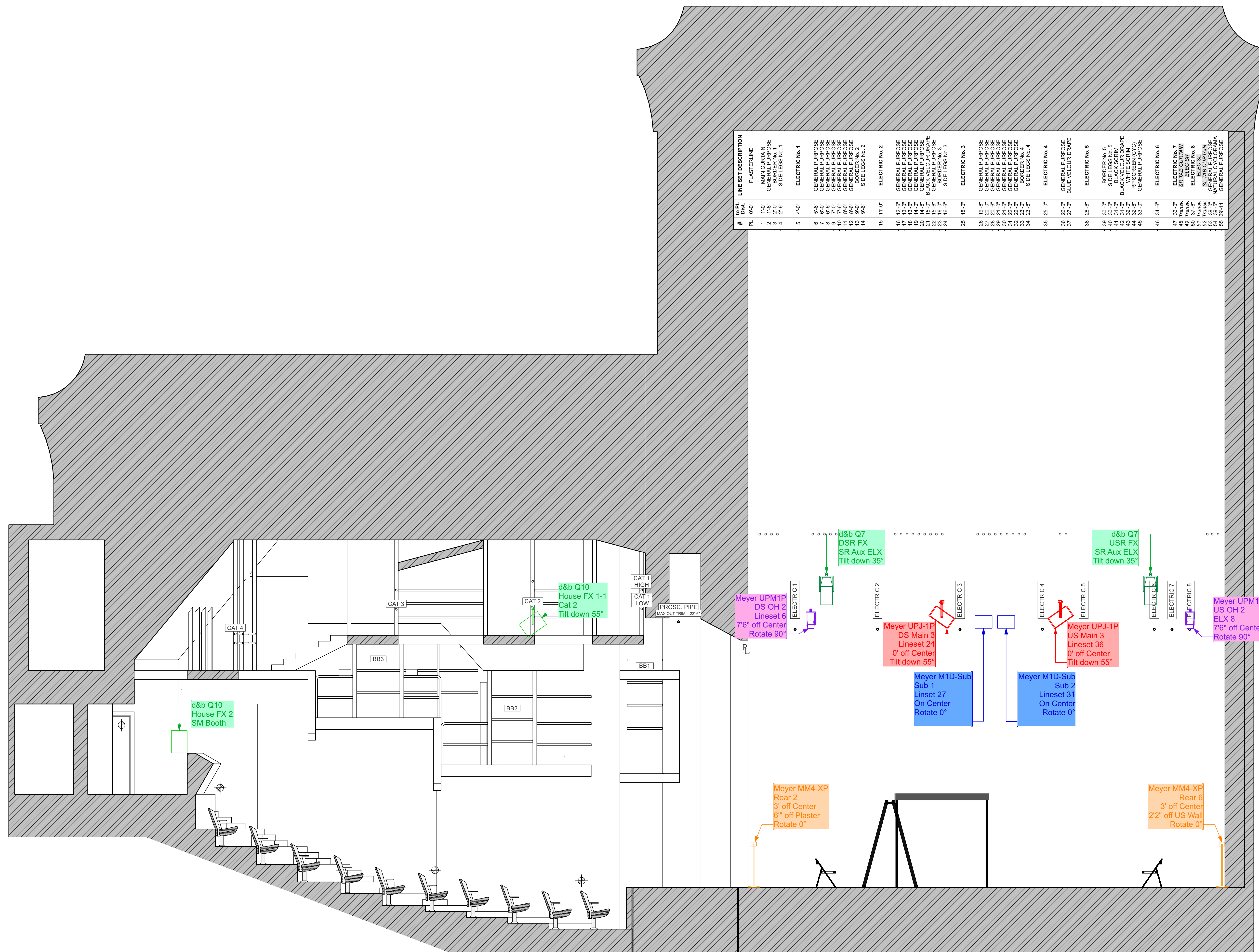
2 Section SR Scale: 1/4" = 1'-0"
